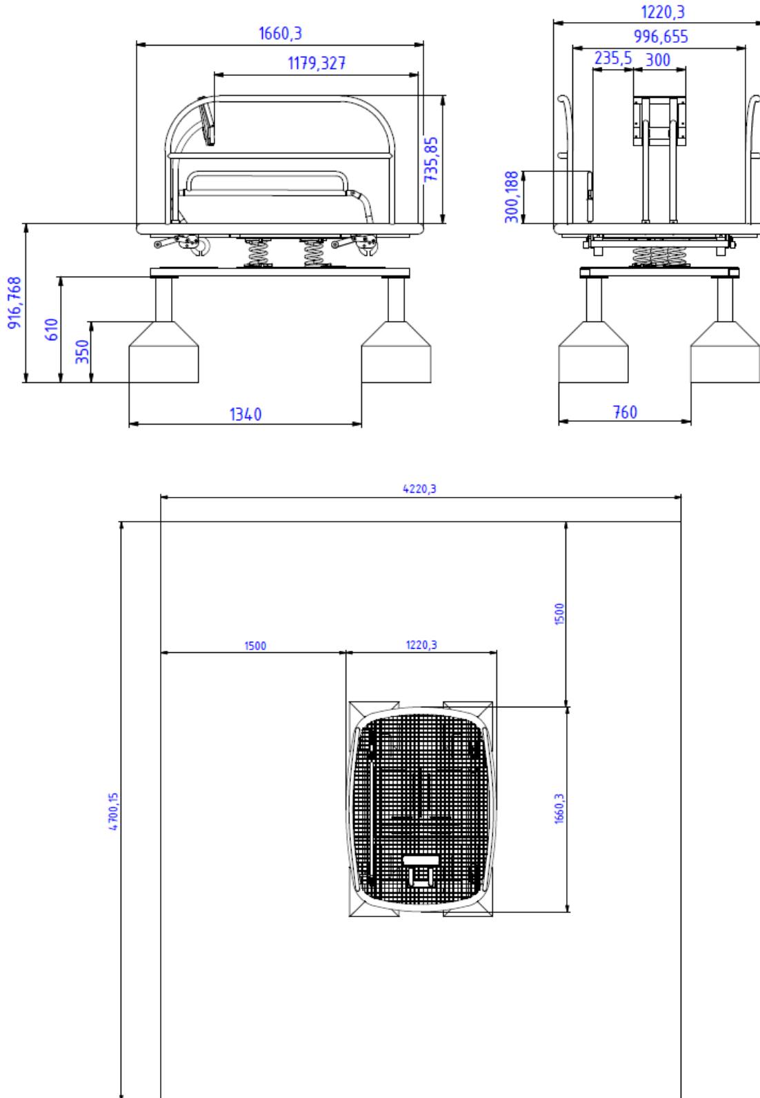
Rys. Wymiary Bujaka integracyjnego TERMA i jego strefy bezpieczeństwa
