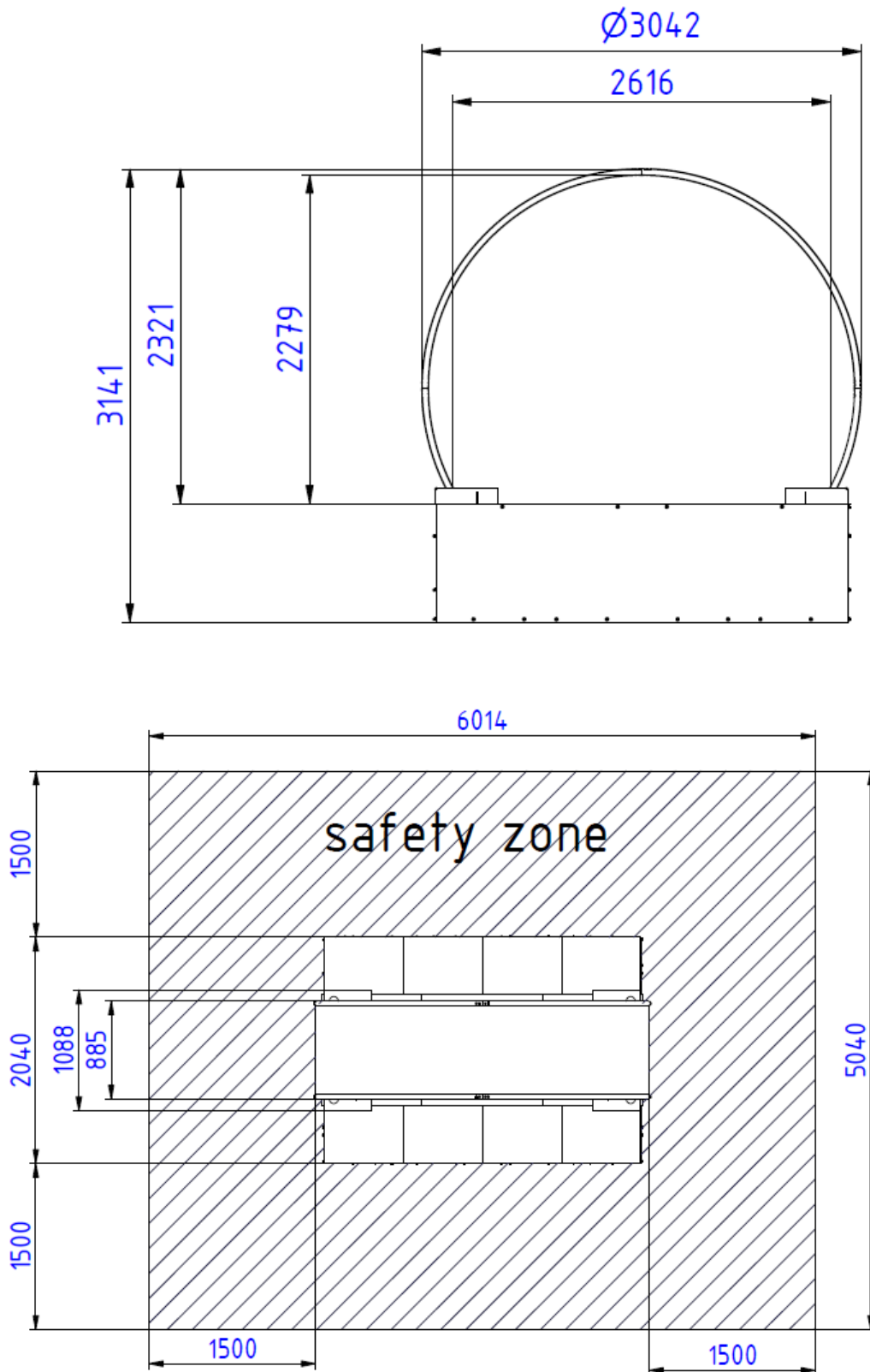
Rys. Wymiary Kołowrotka integracyjnej TERMA i jego strefy bezpieczeństwa.
