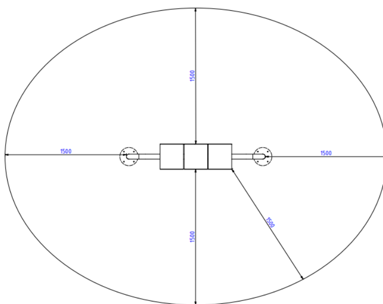
Rys. Wymiary Bloczków integracyjnych poziomych TERMA i strefy bezpieczeństwa
