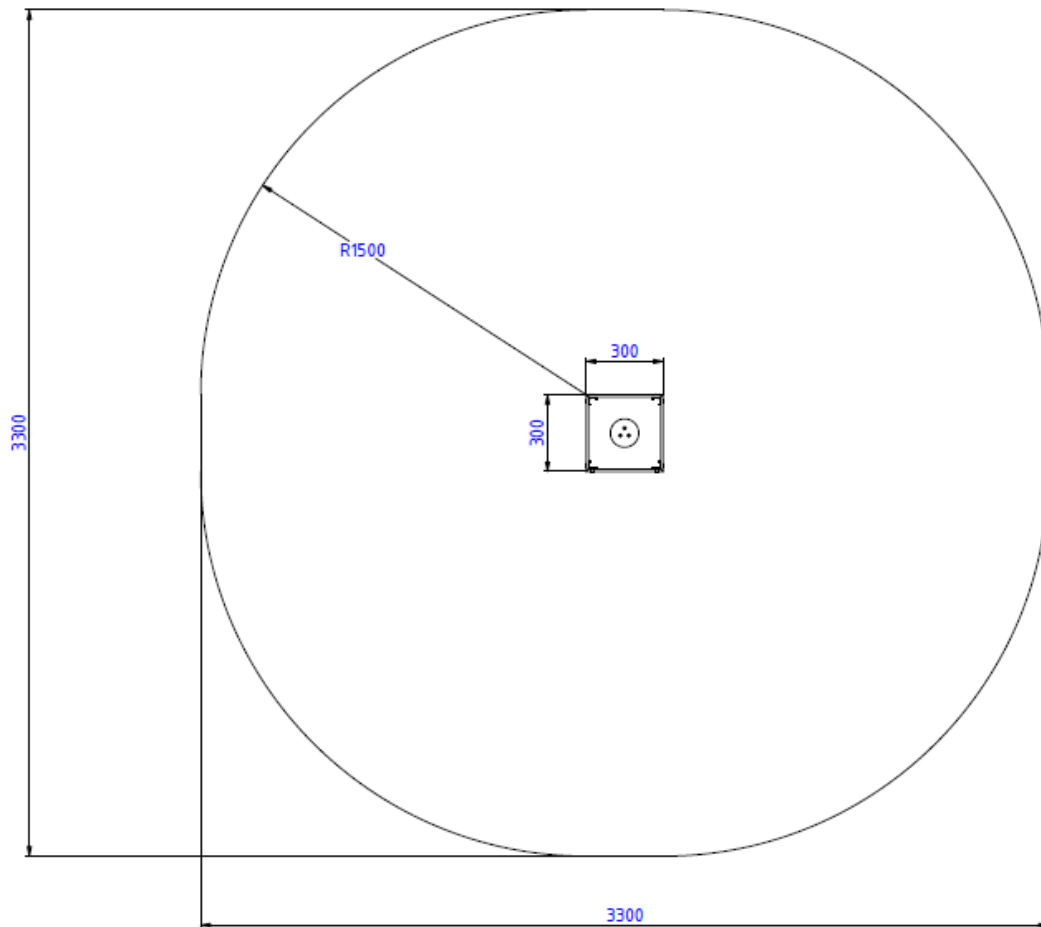
Rys. Wymiary Bloczków integracyjnych TERMA i strefy bezpieczeństwa
