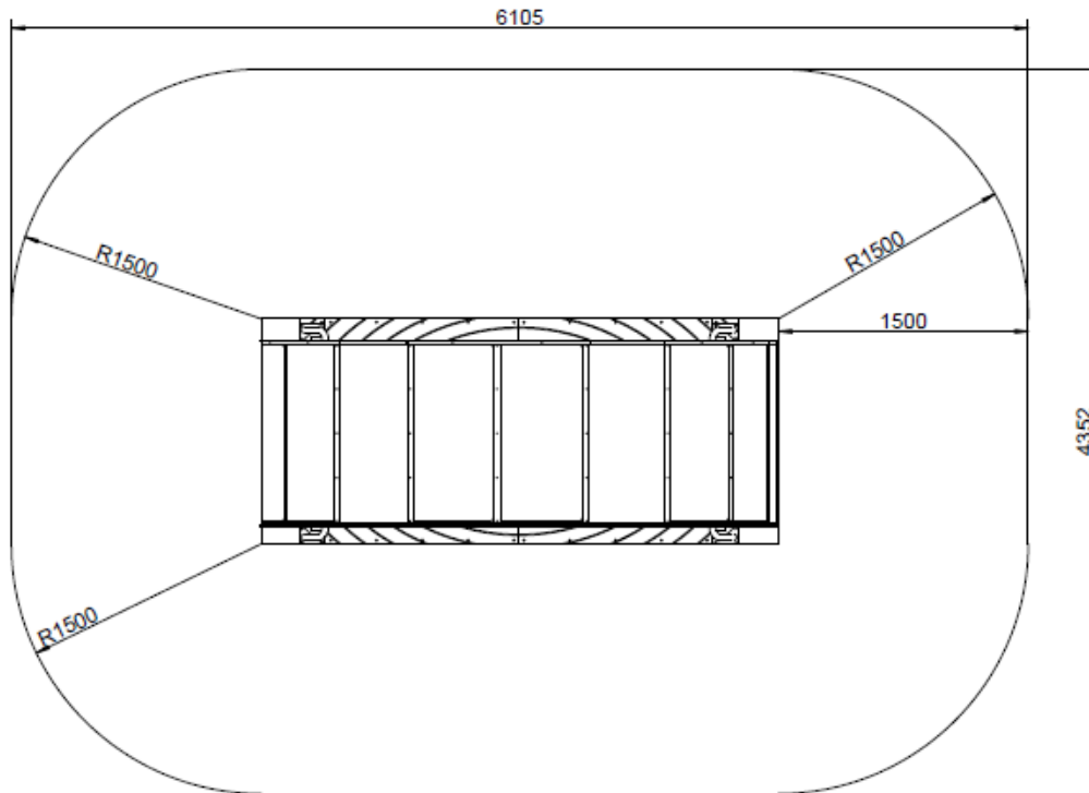
Rys. Wymiary Kołowrotka integracyjnej TERMA i jego strefy bezpieczeństwa.
