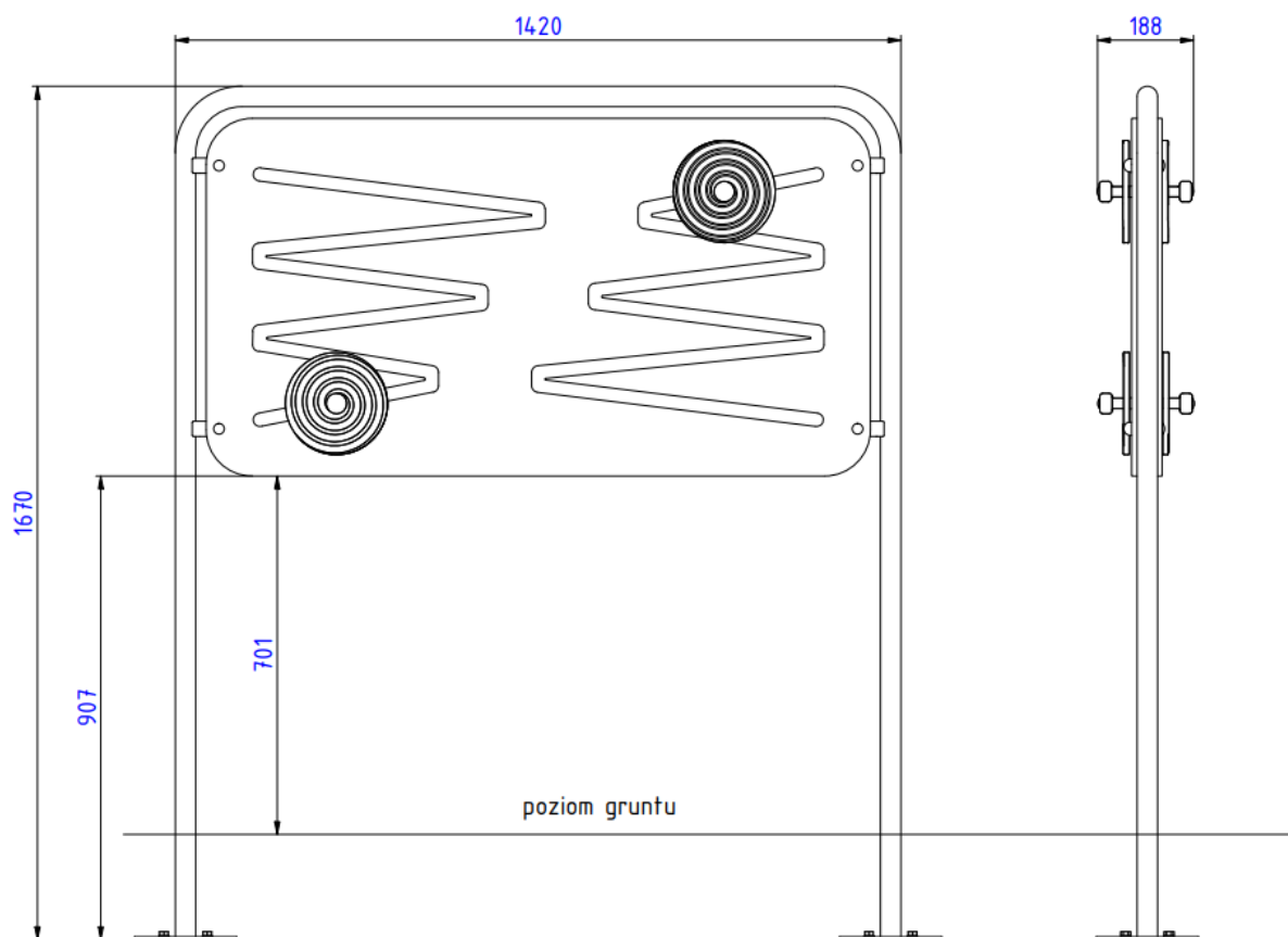
Rys. Wymiary urządzenia
