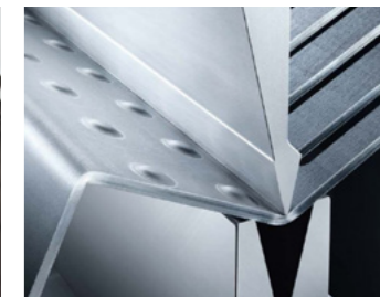
GIĘCIE BLACH NA PRASIE KRAWĘDZIOWEJ
