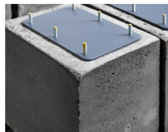
FUNDAMENTY Z CEMENTU PORTLANDZKIEGO KLASY 42,5 R
